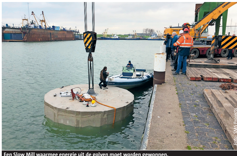
Een Slow Mill waarmee energie uit de golven moet worden gewonnen.
